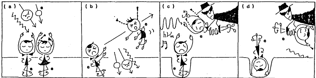
図1. ESR年代測定の原理説明イラスト (a)射線をなすスピン(少年と少女)と自然放射線( \alpha , \beta , \gamma 線), (b)電離, (c)不純物による不対電子の捕獲とマイクロ波の音楽, (d)マイクロ波吸収によるスピンドャンスの逆転, マイクロ波の吸収量から捕獲電子の数, すなわち自然放射線量を求めて, 年代値に換算する。
