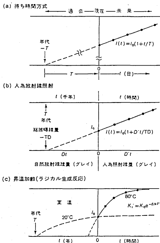
図 1 ESR 年代測定の手法
